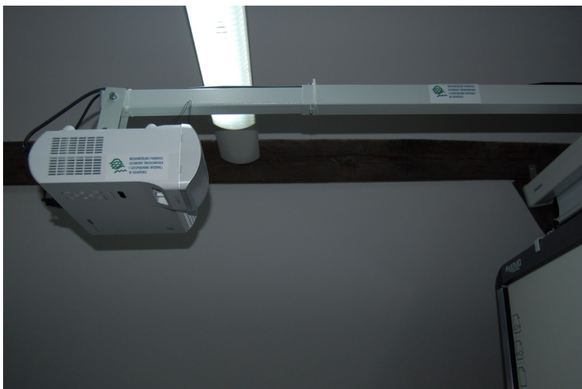
Zestaw interaktywny - tablica interaktywna, projektor krótkoogniskowy, stojak do tablicy i uchwyt do projektora.
